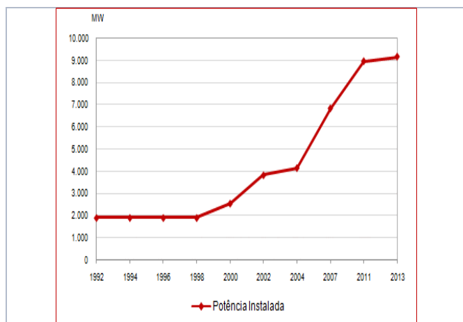
Figura 1: Evolução da potência instalada de geração de energia no RS - 1992 a 2013 (MW) (Fonte: CEEE/Balanco Energético do RS 2012 Aneel Banco de Informações de Geração. Disponível em: www.atlassocioeconomico.rs.gov.br . Acesso em 25 set.2015)
