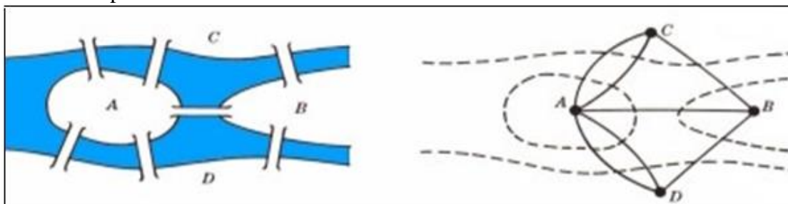
Figura 1 – Euler representou as relações graficamente, associando cada margem da ilha a um nó e a cada ponte um arco.
