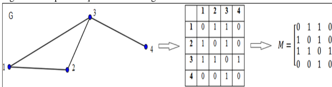
Figura 7 – Representação matricial do grafo G .
