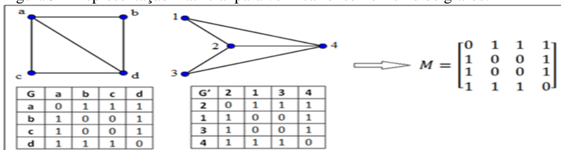
Figura 9 – Representação matricial para verificar o isomorfismo de grafos.
