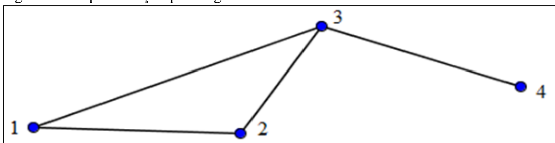
Figura 5 – Representação para o grafo G .
