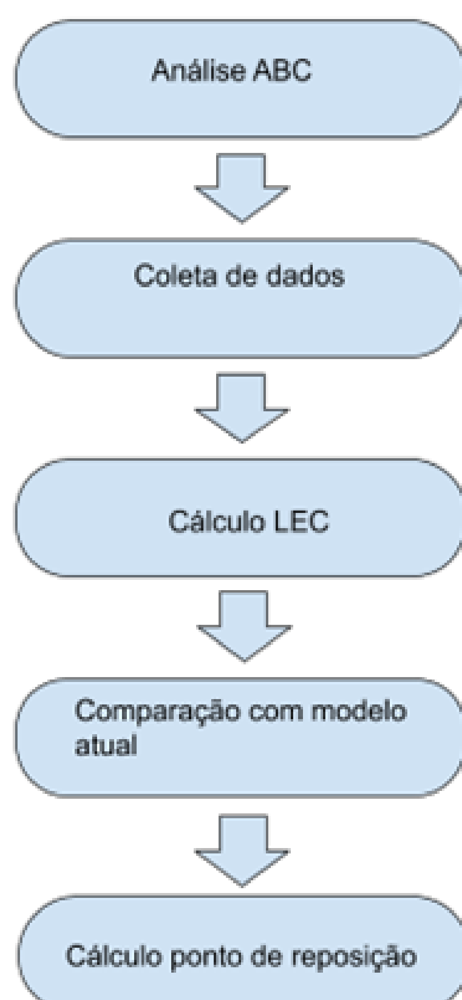
Figura 1 – Macrofluxo do Procedimento Metodológico
